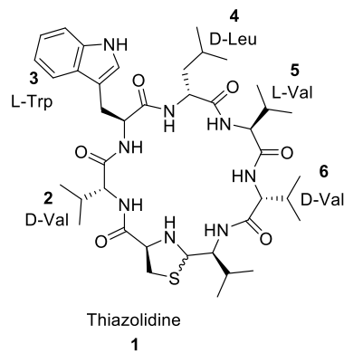
Abbildung 1: Strukturformel Lugdunin
